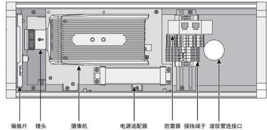
900万AI环保卡口网络摄像机内部结构图：
