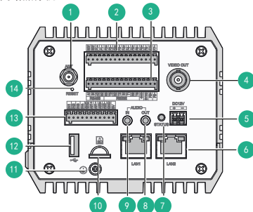
900万AI环保卡口网络摄像机：
